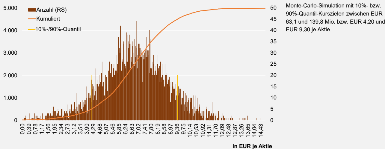
ABBILDUNG 1: HISTOGRAMM DER MONTE CARLO-SIMULATION
