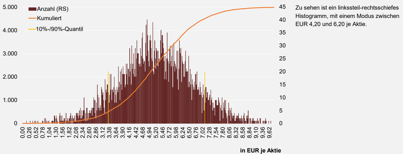
ABBILDUNG 2: HISTOGRAMM DER MONTE CARLO-SIMULATION
